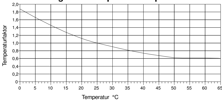
Diagramm Temperaturkompensation
