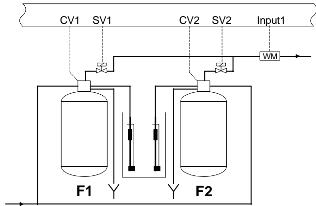
Doppelfilter - Ionenaustauscher
