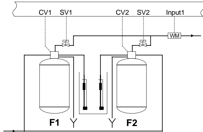
Dubbelfilter – jonbytare
