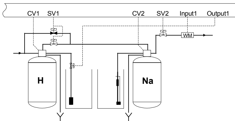
Demineralizzazione parziale a filtro singolo
