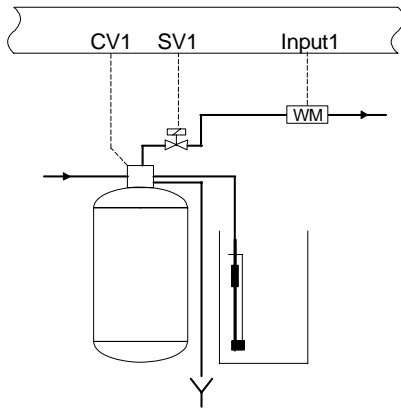
Einfilter – Ionenaustauscher
