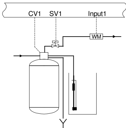
Einfilter – Ionenaustauscher
