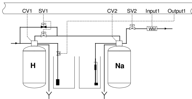
Einstraßen – Teilentsalzung
