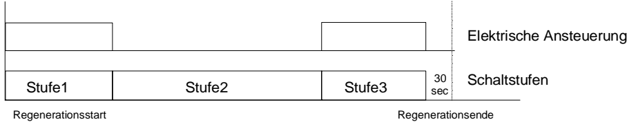
Beispiel 4-Stufenventil mit Nachlaufschaltung
