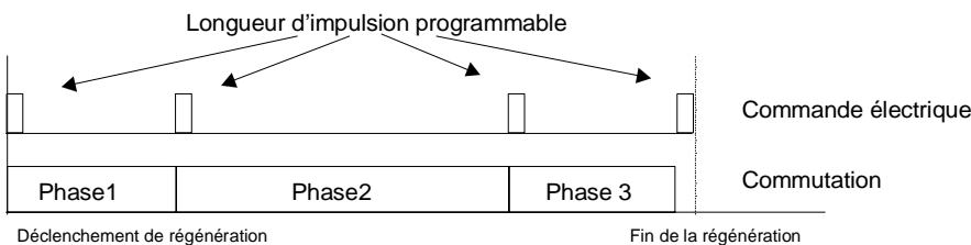
Exemple de vanne à 4 voies avec commutation par impulsions
